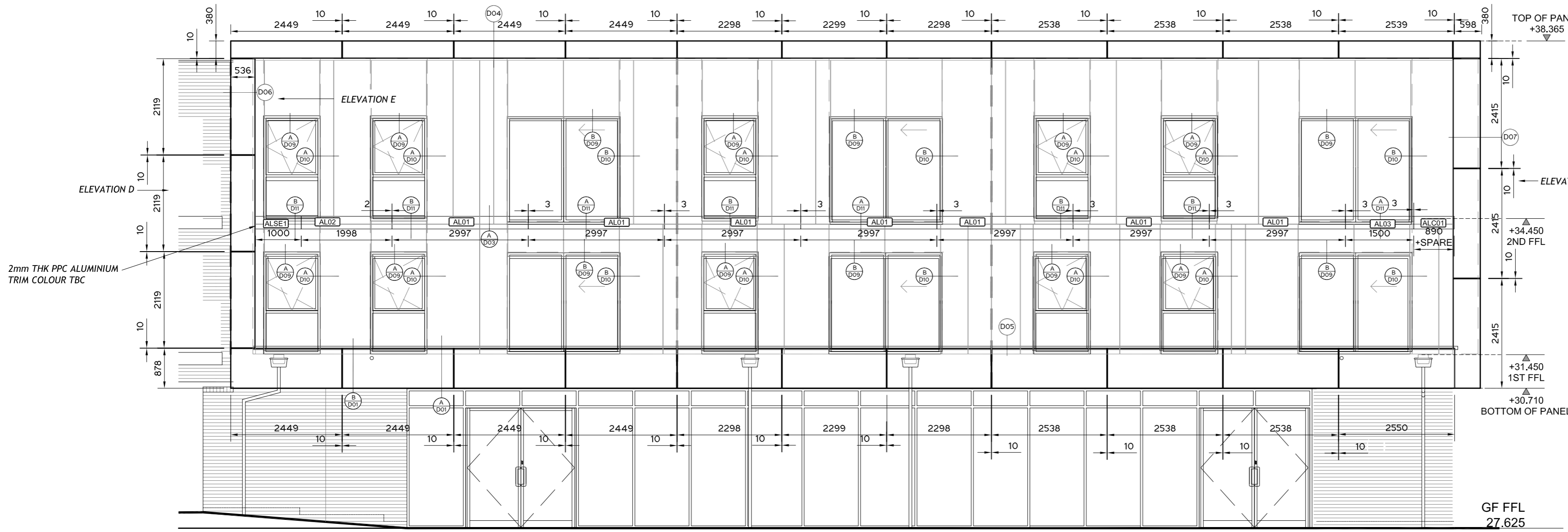
ELEVATION A
